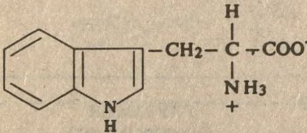
ТРИПТОФАН ( \alpha -амино- \beta -индолилпропи- онова киселина)
