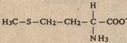
МЕТИОНИН ( \alpha -амино- \gamma -метилтмоас- лена киселина)
